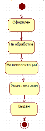
Рис.2 Диаграмма состояний объекта класса Заказ.
