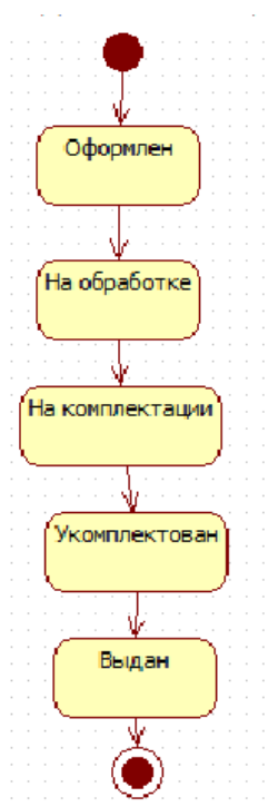
Рис. 2 Диаграмма состояний объекта класса Заказ.
