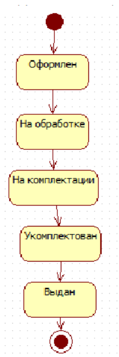
Рис. 2 Диаграмма состояний объекта класса Заказ.
