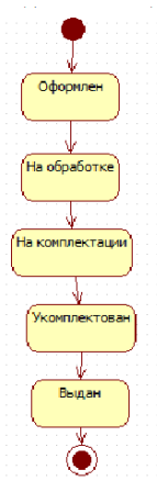
Рис.2 Диаграмма состояний объекта класса Заказ.
