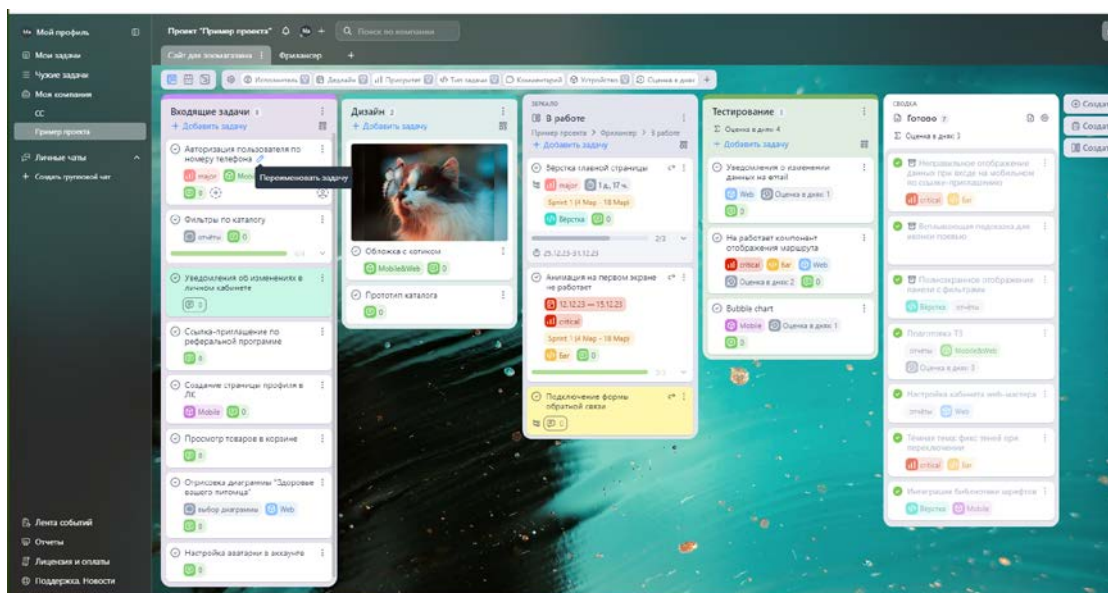
Рис.1 Пример Kanban-доски
